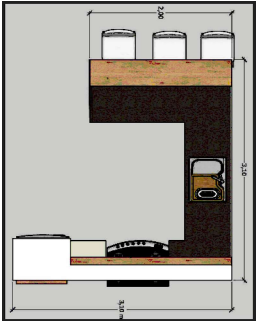
DETALHE COZINHA
